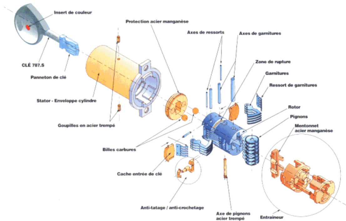
Cylindre éclaté Fichet
